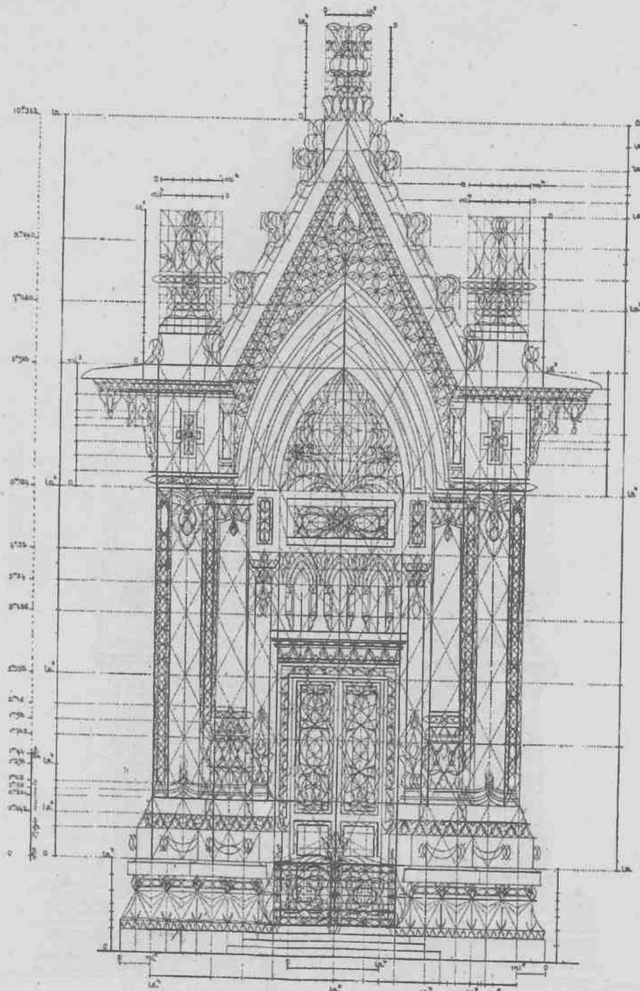
GRANDE CHAPELLE. — Détail du Porche et Porte d'entrée (Style ogival). — Accord La, Ut, Mi.
