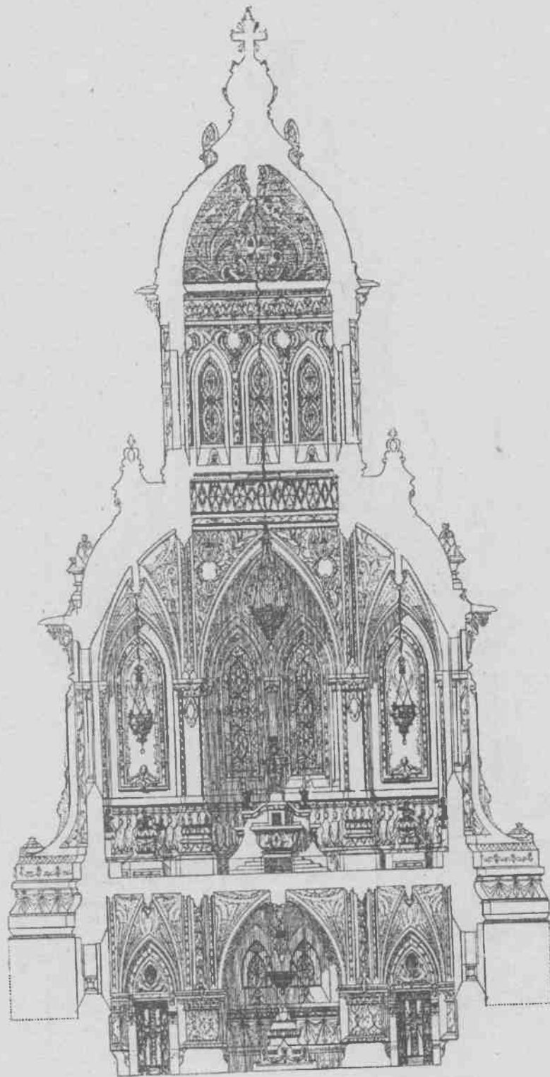
GRANDE CHAPELLE. — Coupe.
