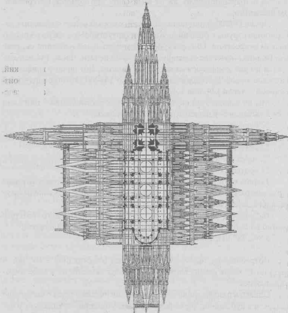
Essai. — Charpente musicale des plan coupes et élévations.
