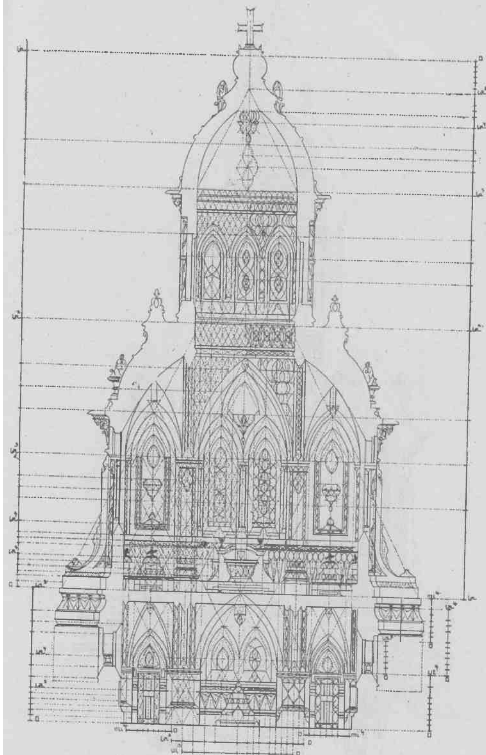
GRANDE CHAPELLE. — Coupe (Style ogival). — Accord La, U, Nl.
