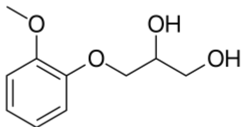
Гвайфенезин
