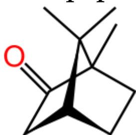
Камфора
