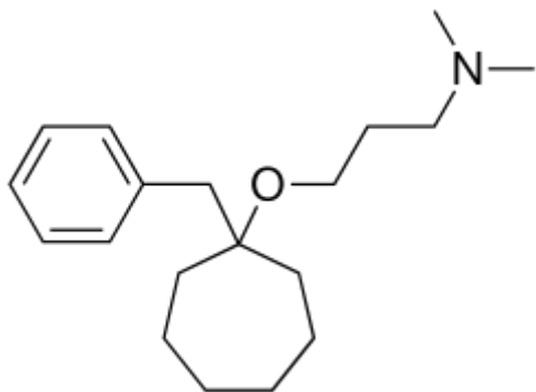
Бенциклан
