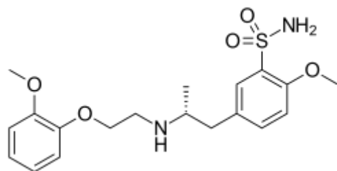
Тамсулозин
