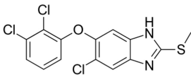
Мебендазол
