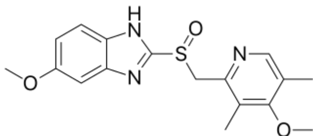
Омепразол
