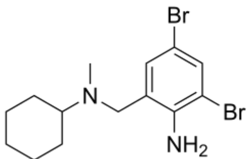
Бромгексин
