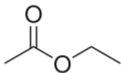
Этилацетат
