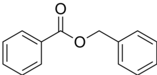
Бензилбензоат
