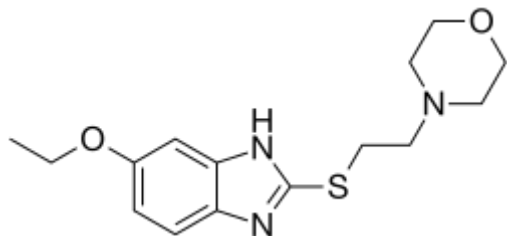
Фабомотизол
