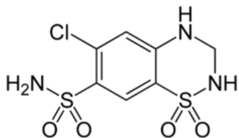
Гидрохлортиазид
