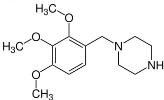
Триметазидин
