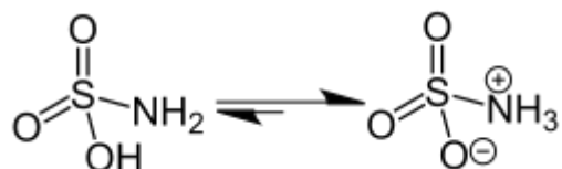
Аминосульфоновая кислота
