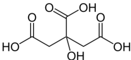
Лимонная кислота
