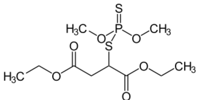
Малатион
