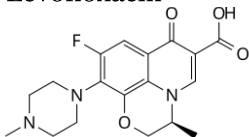
Levofloxacin
