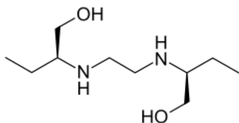
Этамбутол
