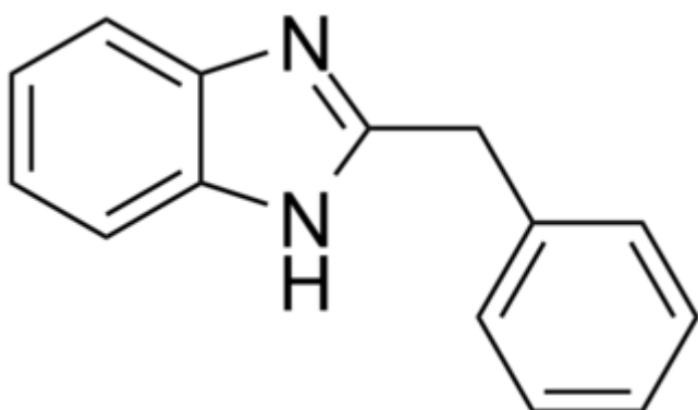
Бендазол
