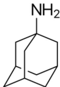
Амантадин
