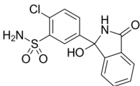
Хлорталидон
