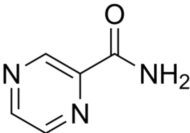
Пираминамид
