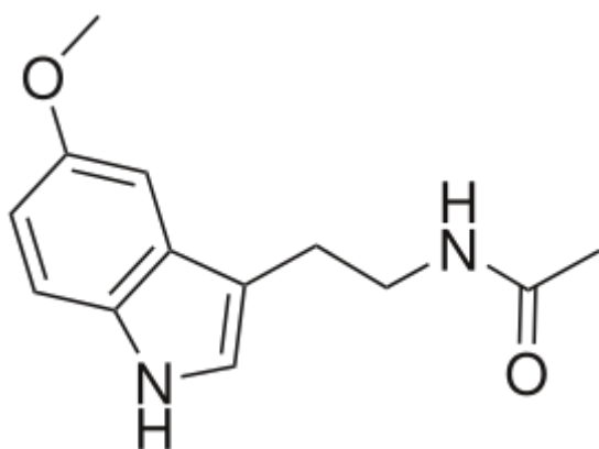
Мелатонин
