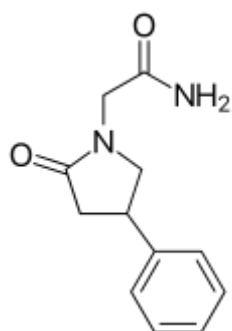
Фонтурацетам
