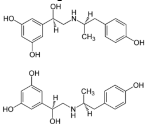
Фенотерол
