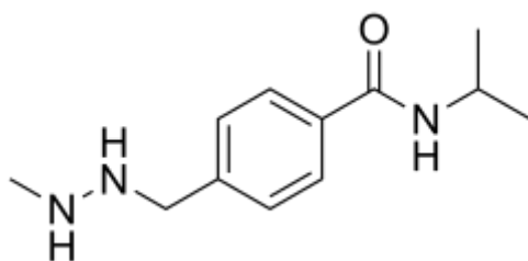
Прокарбазин
