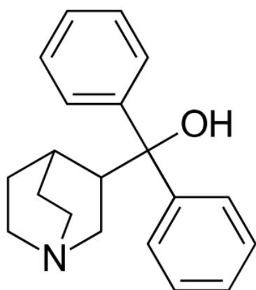
Сехифенадин
