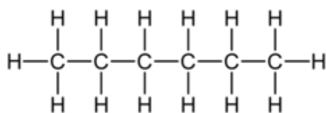
Гексан
