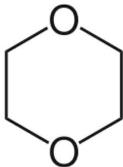
1,4-Диоксан
