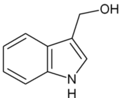
Индол-3-карбинол
