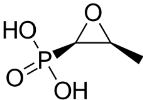
Фосфомицин
