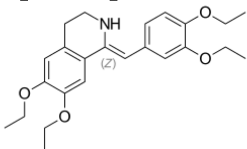
Дротаверин
