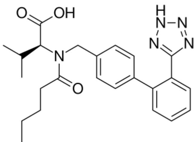
Валсартан
