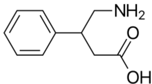
Фенибут
