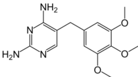
Триметоприм
