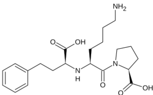
Лизиноприл
