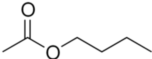
Бутилацетат
