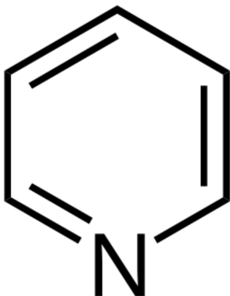
Пиридин
