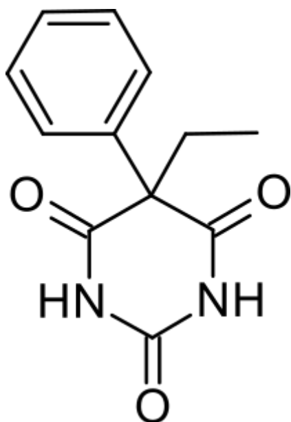
Фенофибрат
