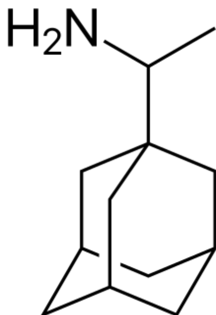
Римантадин
