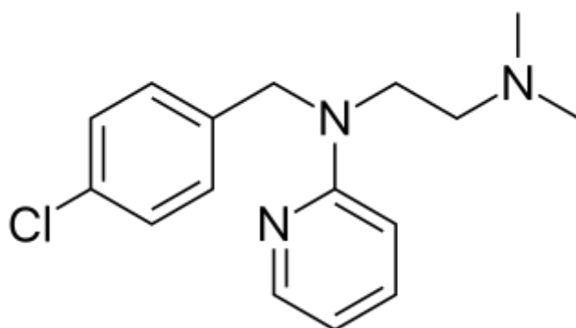
Хлоропирамин
