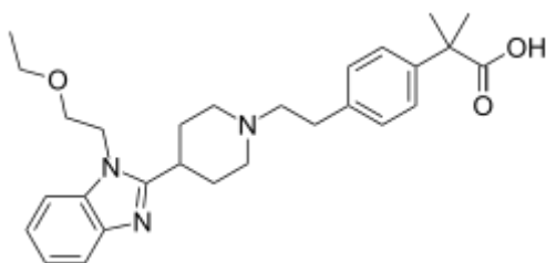
Биластин
