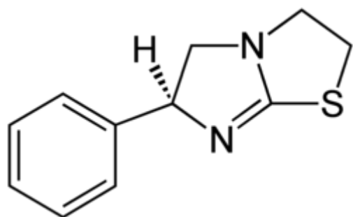
Левамизол
