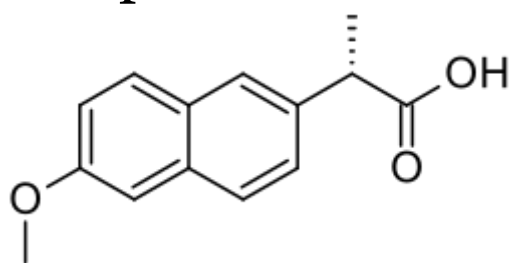
Напроксен
