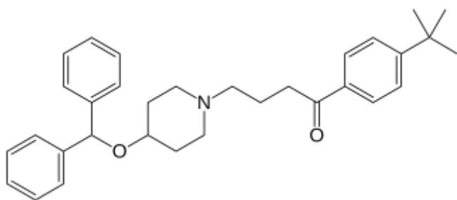
Эбастин
