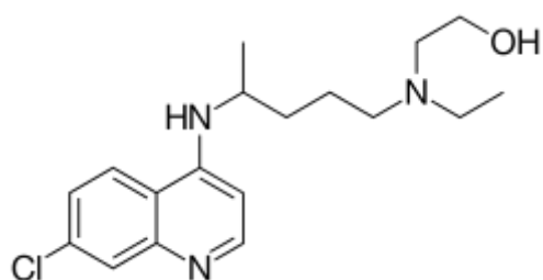
Гидроксихлорохин
