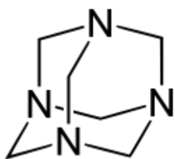
Уротропин
