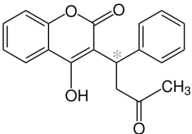
Вилдаглиптин
