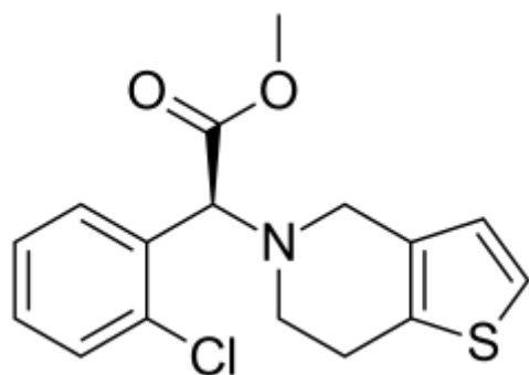
Клопидогрел
