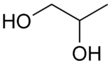
Пропиленгликоль
