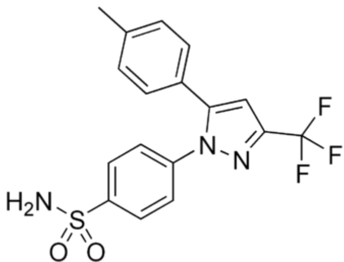
Цефалотин
