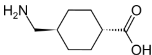
Транексамовая кислота
