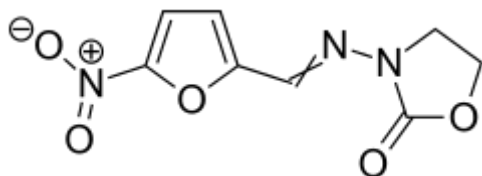
Фуразолидон
