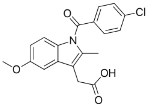
Индометацин
