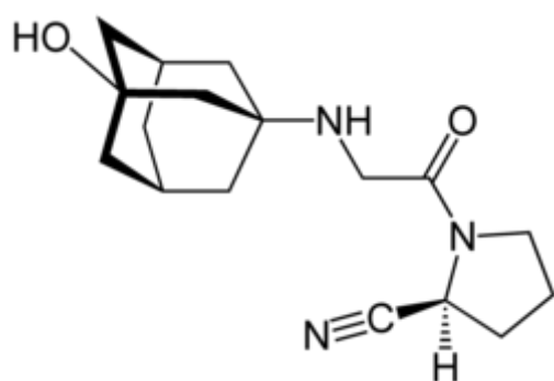
Вилдаглиптин
