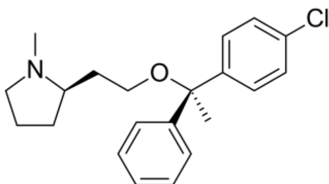
Клемастин
