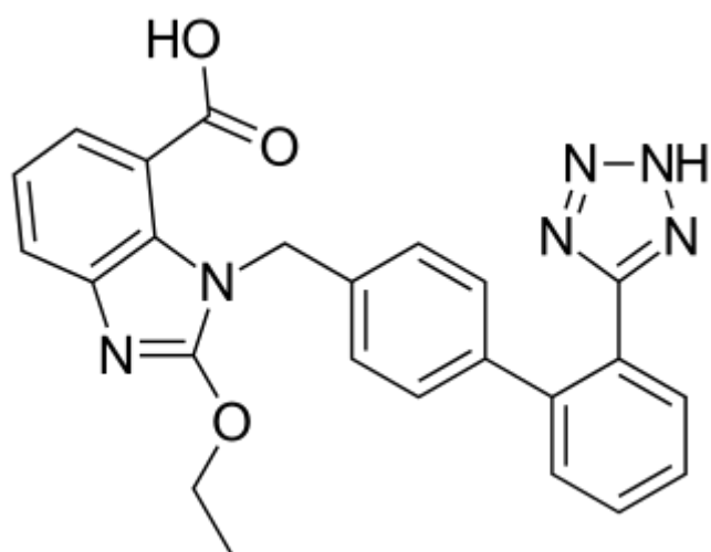
Кандесартан
