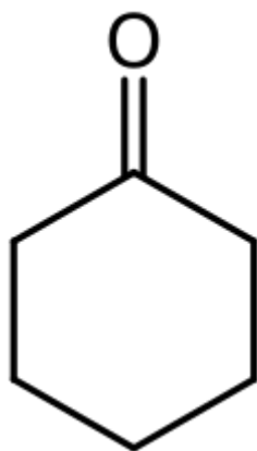
Циклогексанон
