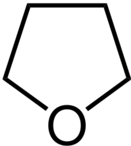
Тетрагидрофуран
