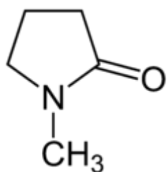
N -Метил-2-пирролидон
