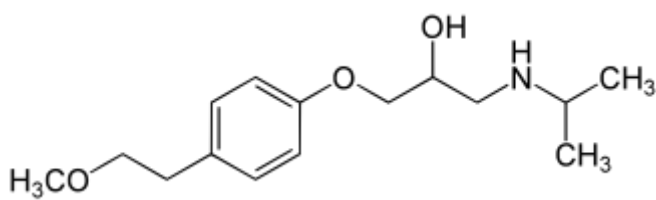
Метопролол
