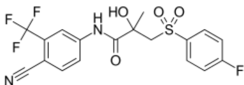
Бикалутамид
