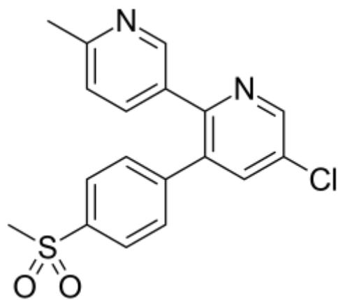
Эторикоксиб
