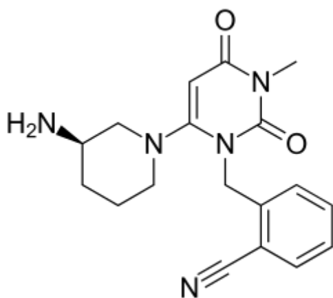
Алоглиптин
