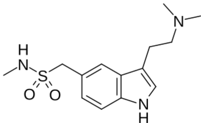
Суматриптан
