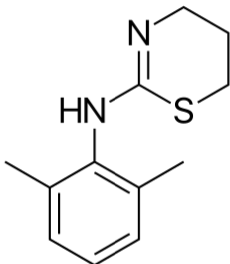
Ксилазин
