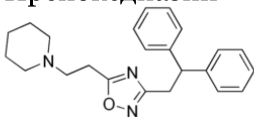
Преноксидиазин
