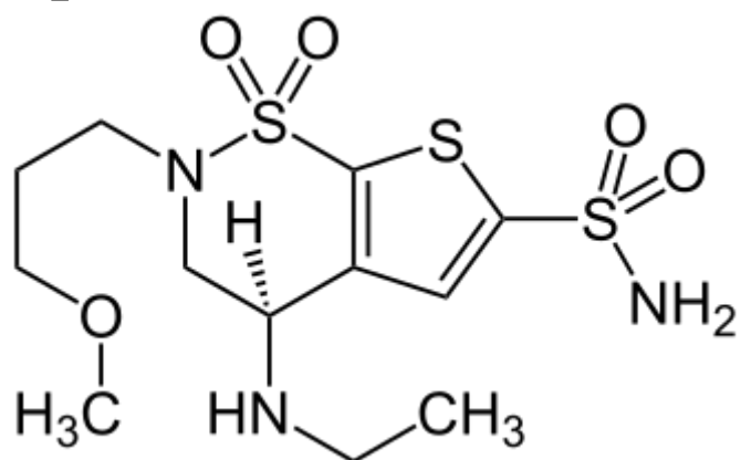
Бринзоламид
