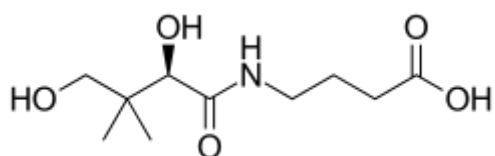
Гопантенная кислота
