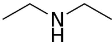
Диэтиламин
