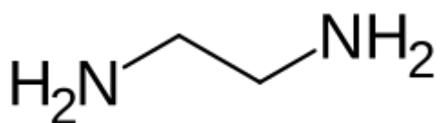
Этилендиамин
