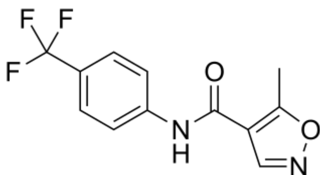
Лефлуномид
