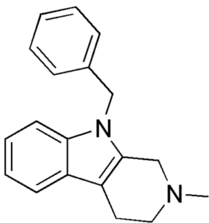
Доксиламин
