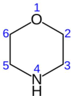
Морфолин
