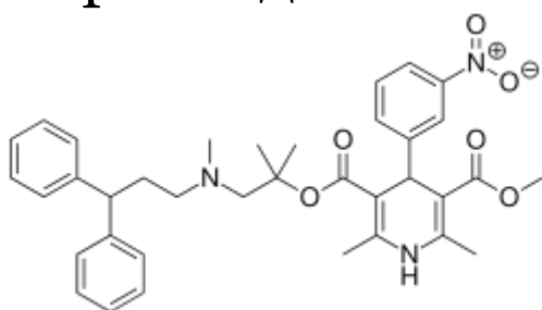
Лерканидипин
