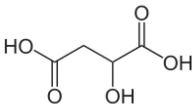
Яблочная кислота
