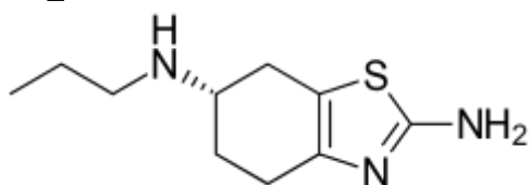
Прамипексол
