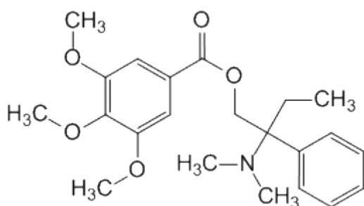
Тримебутин
