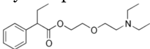
Бутамират
