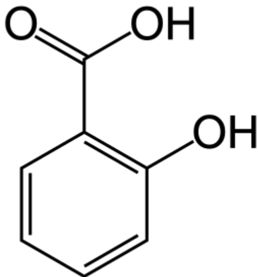
Салициловая кислота
