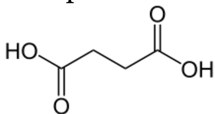
Янтарная кислота
