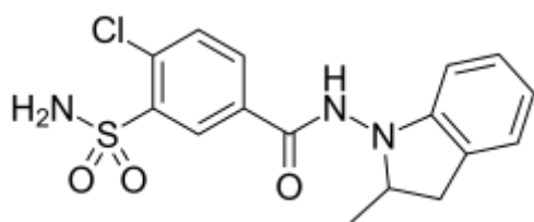
Индапамид
