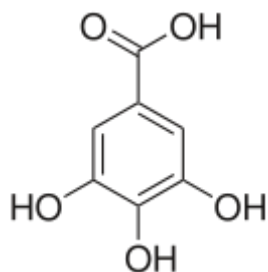
Галловая кислота
