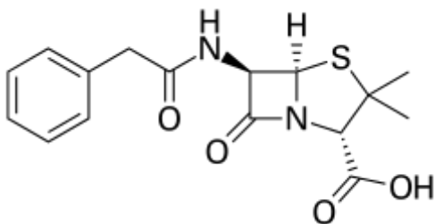
Бензилпенициллин
