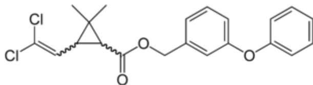
Перметрин
