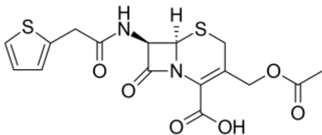
Цефалотин
