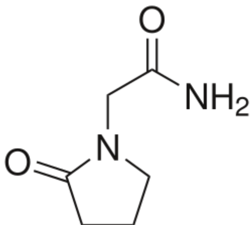
Пирацетам
