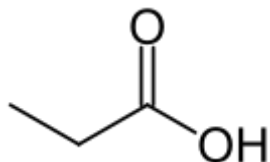
Пропионовая кислота
