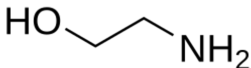
Этаноламин
