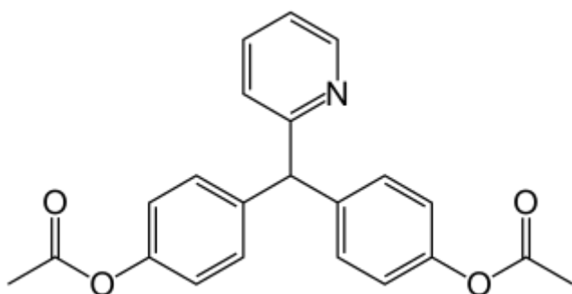
Бисакодил
