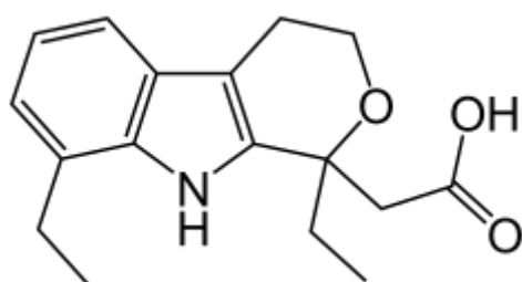
Этодолак
