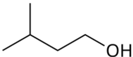
Изоамиловый спирт
