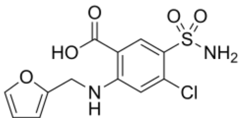
Фуросемид
