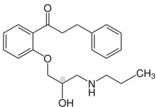
Пропафенон
