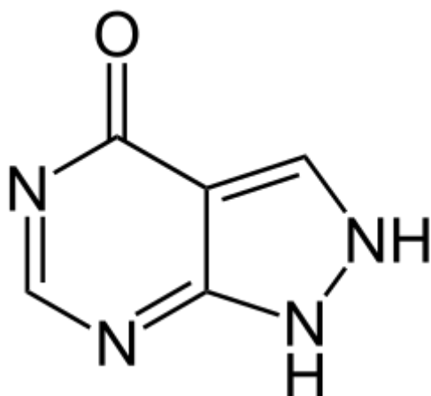
Алоглиптин
