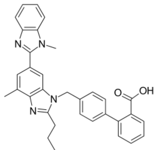
Телмисартан
