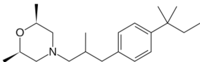
Аморолфин
