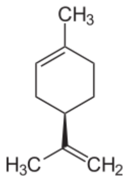
Лимонен
